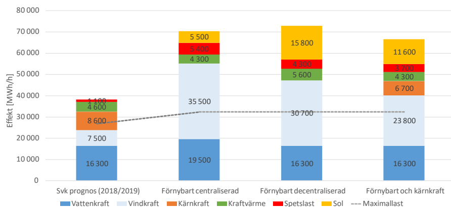
Figur: Tre olika scenarier för 100% fossilfri elproduktion i Sverige år 2045, som analyserats i studien. Figuren anger den installerade produktionskapaciteten
