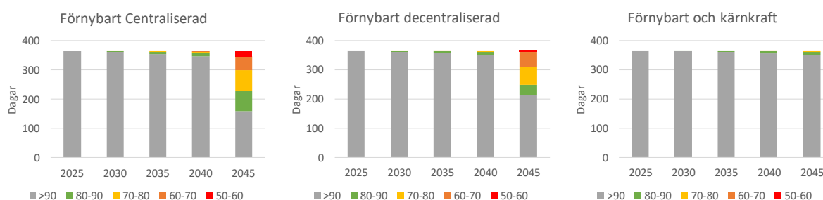
Figur 24: Antal dagar med lägre svängmassa än motsvarande 90 GWs.
