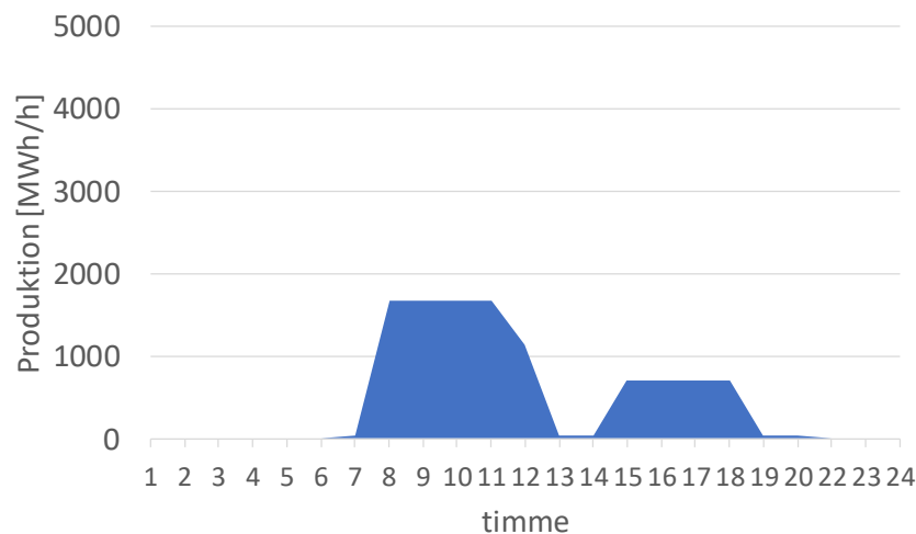
Figur 40 Spetslastproduktion jan-mars en 20-års vinter, scenariot "Förnybart centraliserad"
