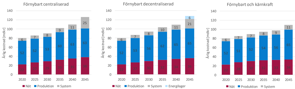
Figur 14: Utveckling systemkostnad fördelat på nät, produktion & systemtjänster
