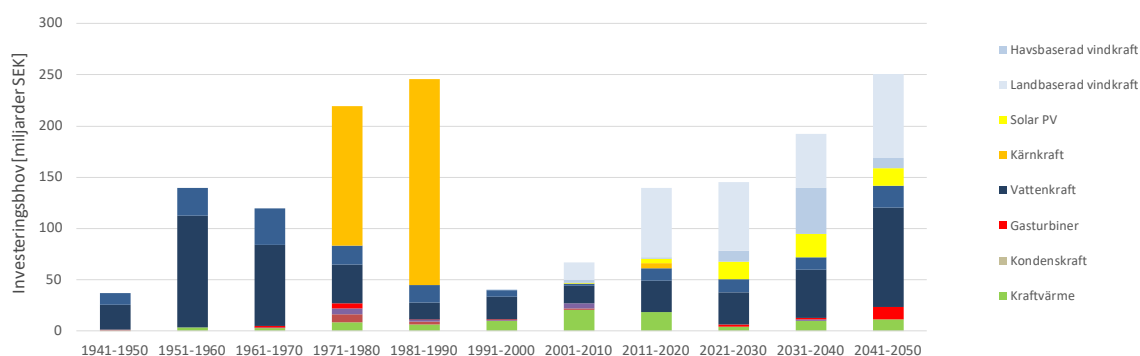
Figur 17: Investeringar i kraftproduktion i scenariot ”Förnybart centraliserad” i ett historiskt perspektiv
