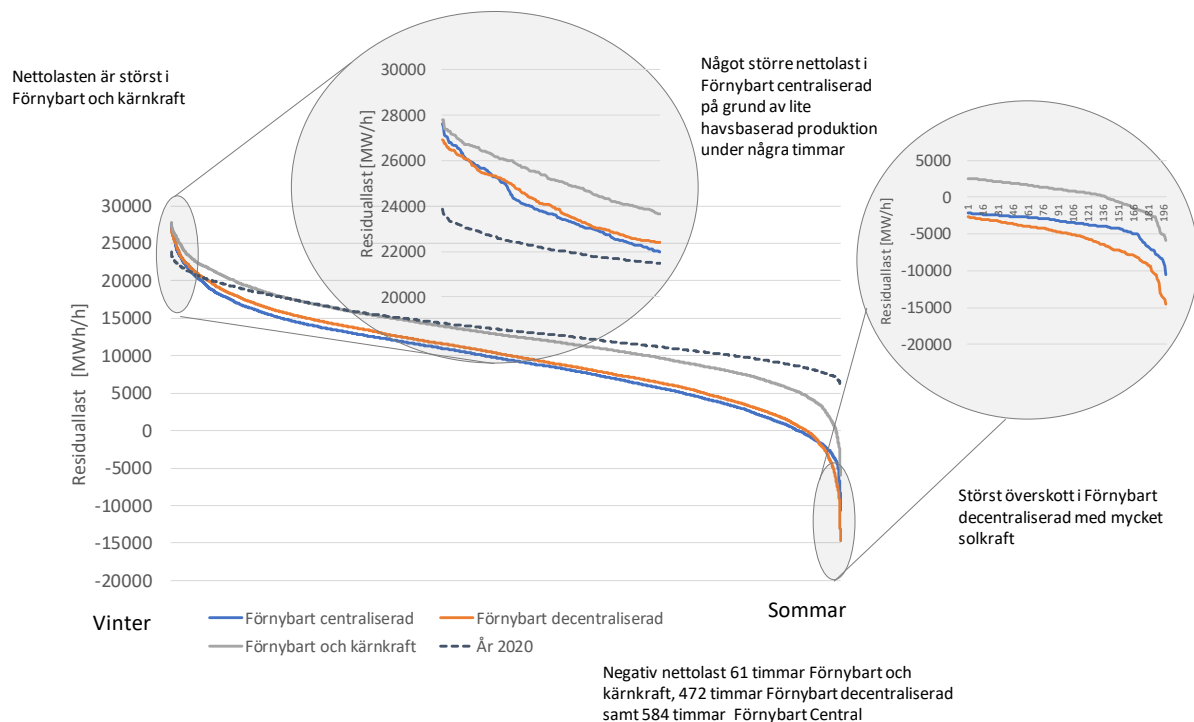
Figur 52: Nettolasten för de tre scenarierna år 2045
