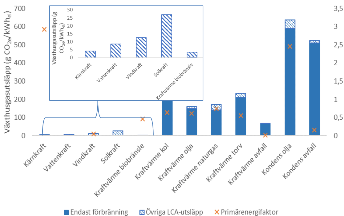
Figur 33. Emissionsfaktorer och primärenergifaktorer för olika kraftslag.
