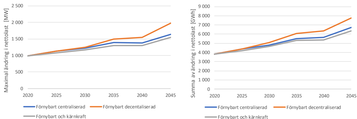
Figur 27: Ändringar i nettolast. Till vänster maximal skillnad från en timme till nästa (90:e percentilen). Till höger summerad ändring i nettolast för respektive år.
