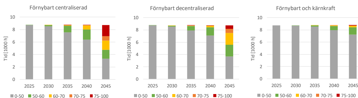
Figur 26: SNSP i olika scenarier
