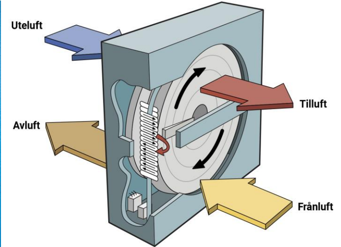
FTX-ventilation
